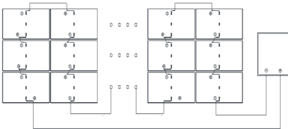
图 9-4 长线缆组件的水平安装方式
