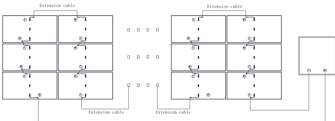
图 9-2 短线缆组件的水平安装方式
