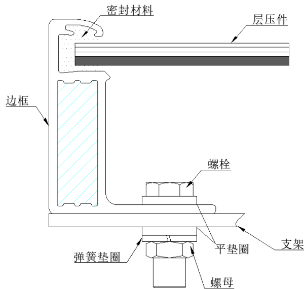
图 8-1 螺栓安装示意图
