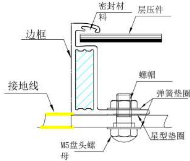
图 11-1 M5 盘头螺钉接地示意图
