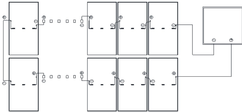
图 9-3 长线缆组件的垂直安装方式
